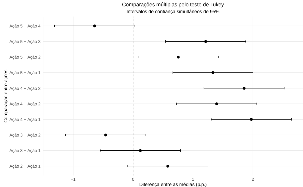
Figura 4: Comparações múltiplas pelo teste de Tukey: intervalos de confiança simultâneos de 95% (em pontos percentuais)
