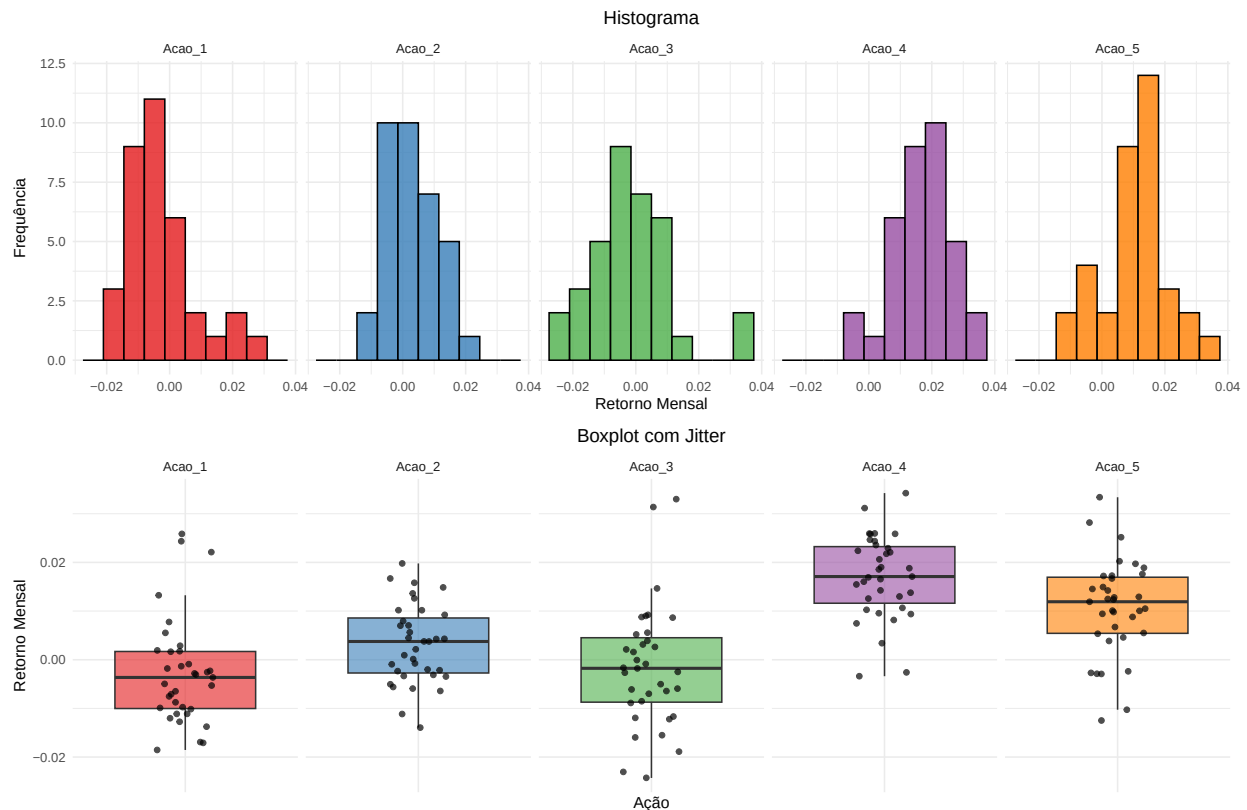
Figura 1: Comparação das distribuições dos retornos mensais: Histograma e Boxplot com Jitter
